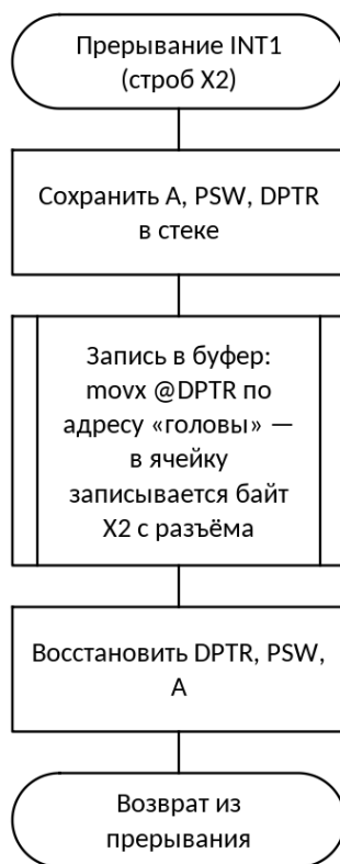
Рисунок 6 — Схема алгоритма: Обработчик прерывания INT1: приём отсчёта X2 от внешнего устройства
